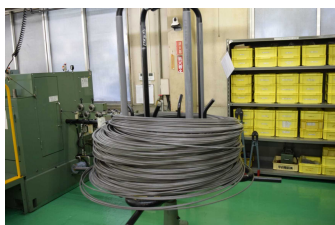
材料 (冷間圧造用炭素鋼線)
